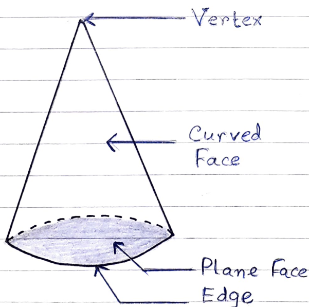
Cone
